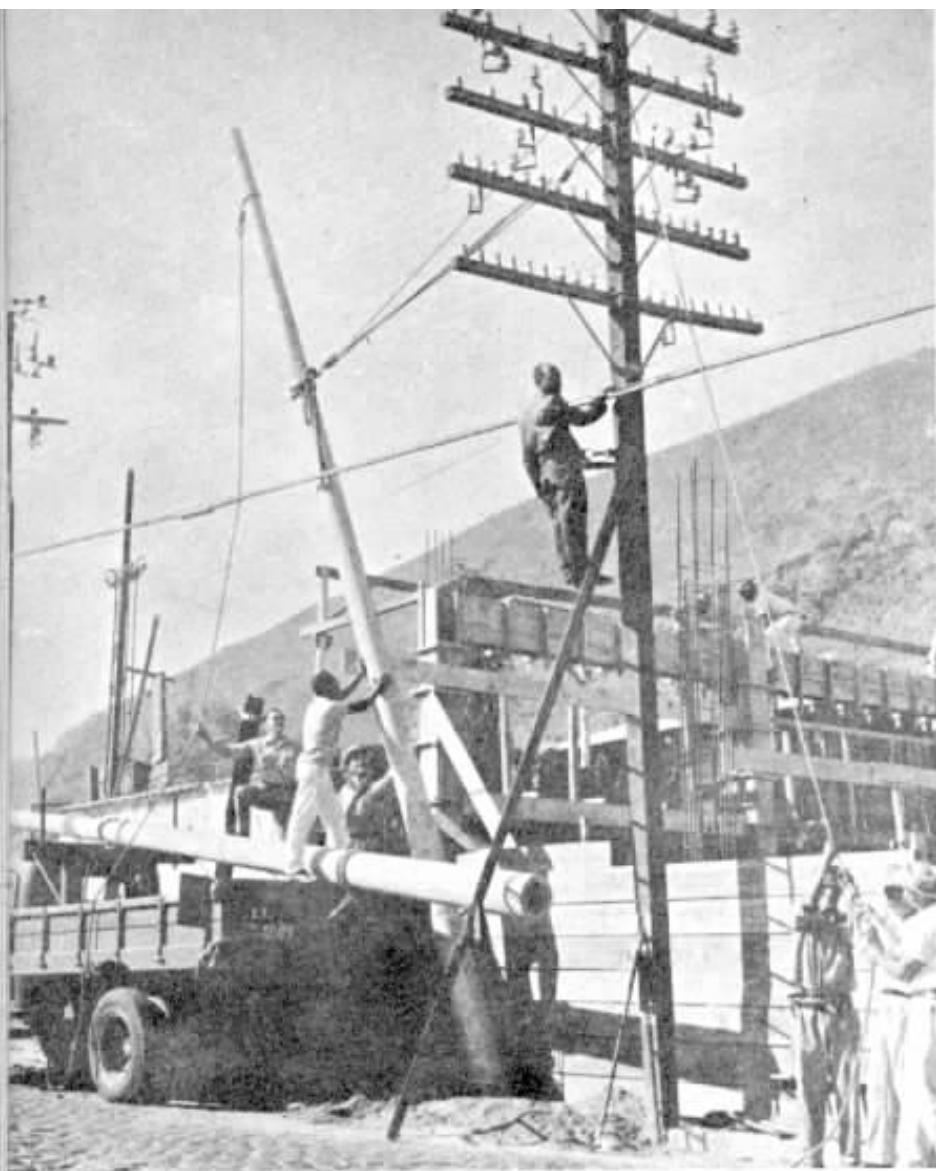
A entrada de Barra Mansa, Oswaldo, Odair, José, Afonso, Expedito, Geraldo e Antonio, num trabalho coordenado, substituem um poste de ferro por outro de cimento armado. O caminhão, de marcha a ré, ajuda a colocá-lo no lugar.
