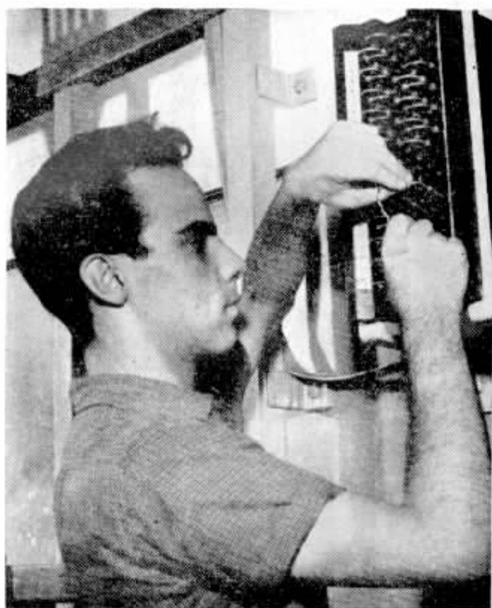
Acima, o conservador Vicente de Paula Libonatti, colocando em seu lugar, um comutador de equipamento 2-VF, das ligações interurbanas de Petrópolis. Abaixo, o conservador Francisco Assis dos Reis, da cidade das hortências, examinando o terminal do cabo coaxial.
