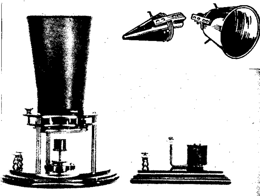
Transmissor e receptor do telefone de Bell que serviram para transmissão do primeiro recado em 10 de Março de 1876. Em cima o telefone patenteado em 7 de Março de 1876.
