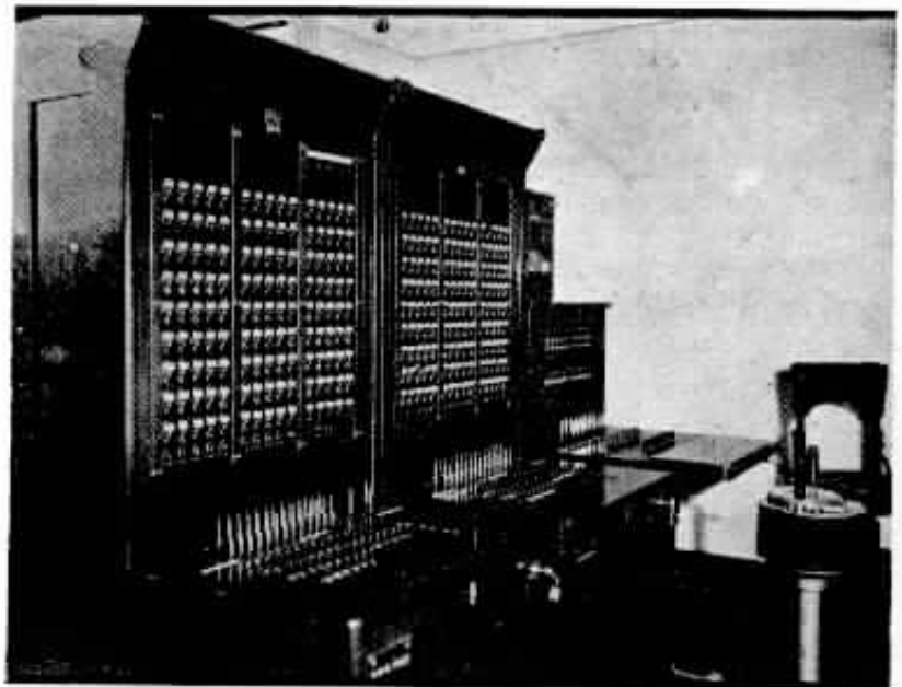
A nova mesa de ligações, que possui duas posições locais e uma interurbana.
