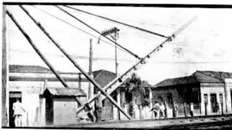
Poste de concreto armado, tipo "Cavan" de 18,20 metros, ao ser levantado em Osasco.
