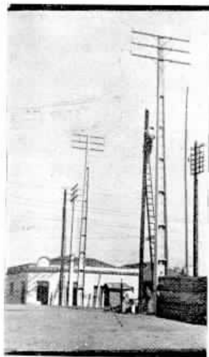
Poste de concreto armado, tipo "Cavan" de 18,20 metros, ao ser levantado em Osasco.
