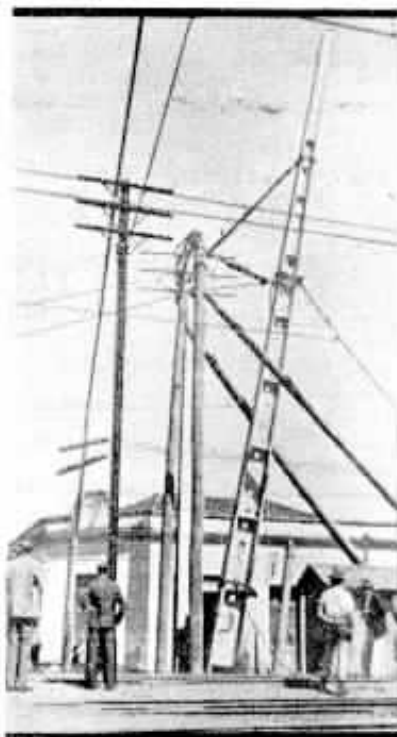
Poste de concreto armado, tipo "Cavan", de 18,20 metros, ao ser levantado em Osasco.
