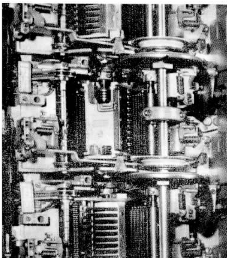
Buscador de chamada de uma estação automática.
