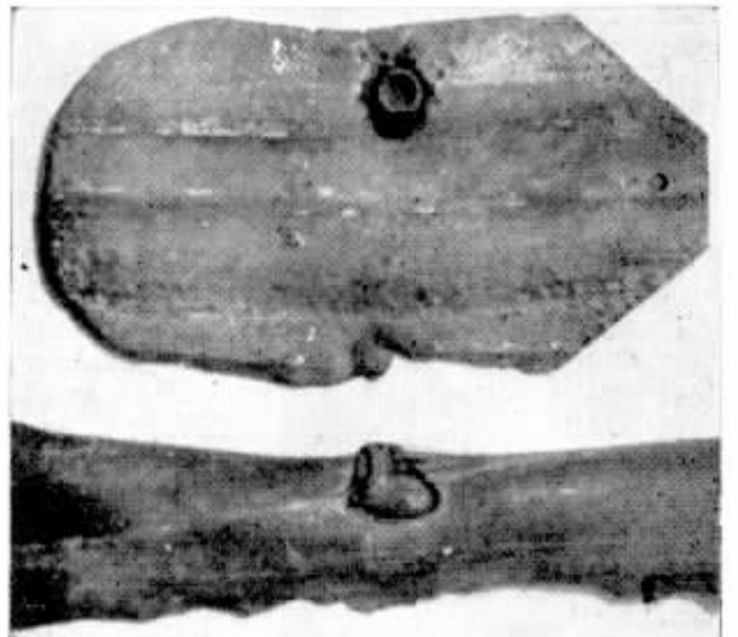
Balas de revólver, encravadas no chumbo de revestimento dos cabos. Fato responsável por sérias interrupções nas ligações. Abaixo, uma raiz de árvore que, caprichosamente, rompeu uma galeria de dutos, enlaçando o cabo.
