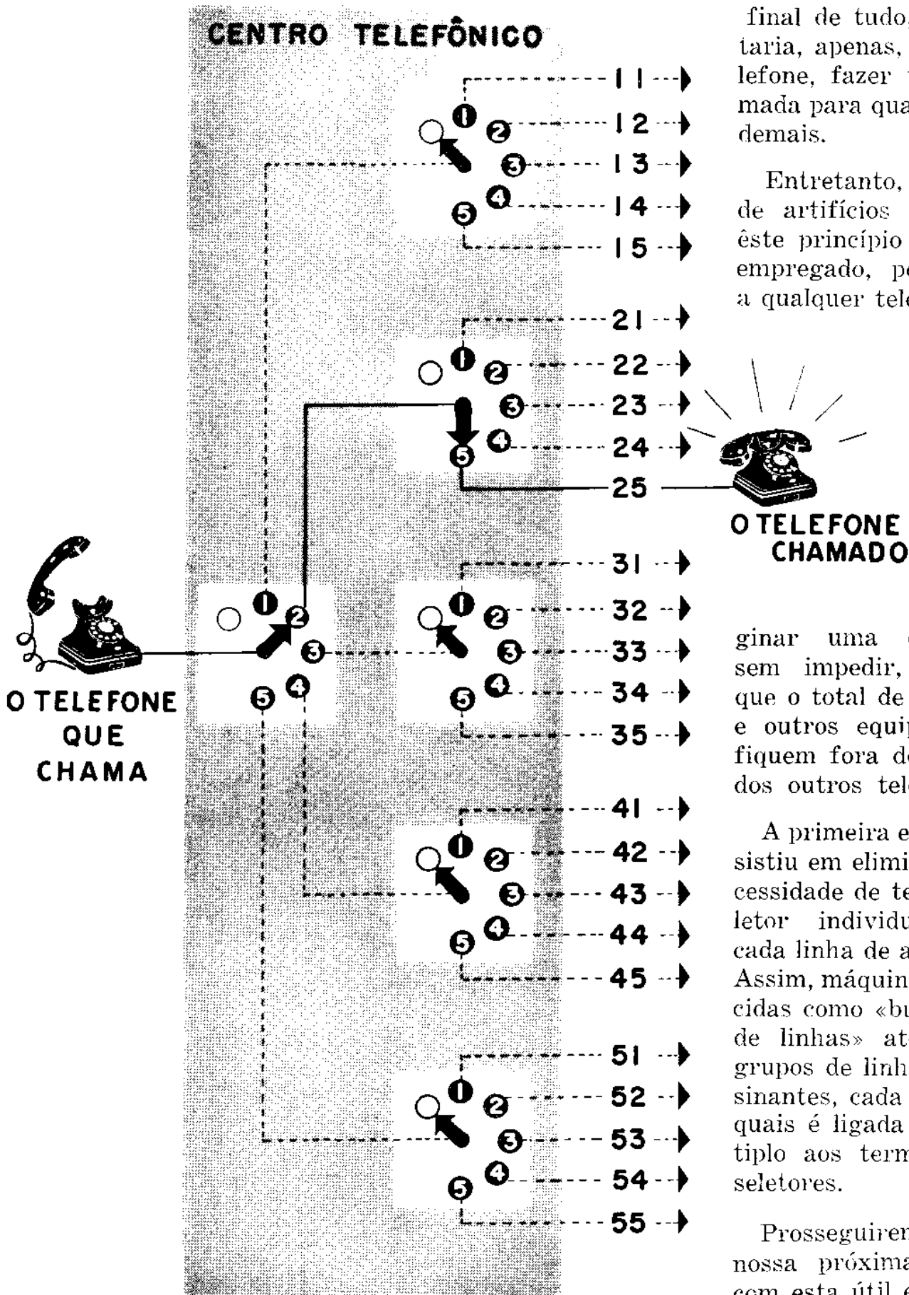
O desenho dá uma idéia do processamento de uma chamada pelo sistema automático. A operação é controlada pelo disco do aparelho que chama e que transmite impulsos elétricos a distância, correspondendo o número de impulsos ao algarismo discado.
