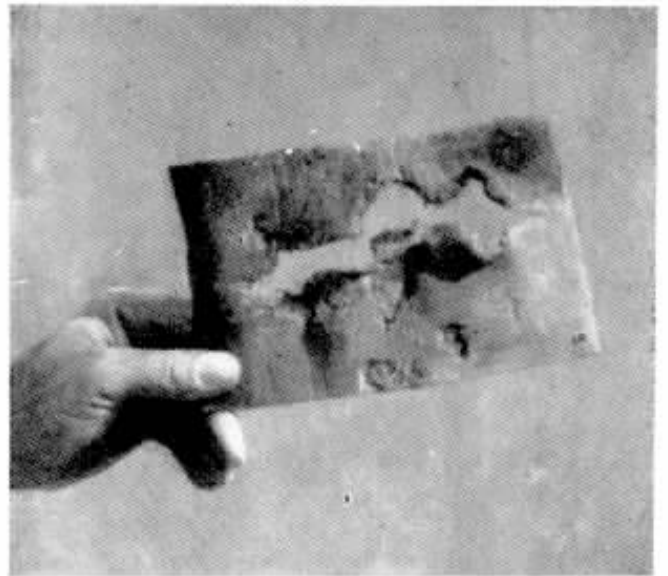
Esta foto dá bem uma idéia dos efeitos da corrosão química ou eletrólise sobre a capa de chumbo dos cabos. Outro sério inimigo, este.
