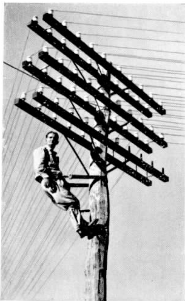
A escada é auxiliar indispensável ao guarda-fios. Junto a pontes de trilho, ferro tubular ou de cimento, é essencial. Nos postes de madeira, a espora de ponta aguçada, também resolve.
