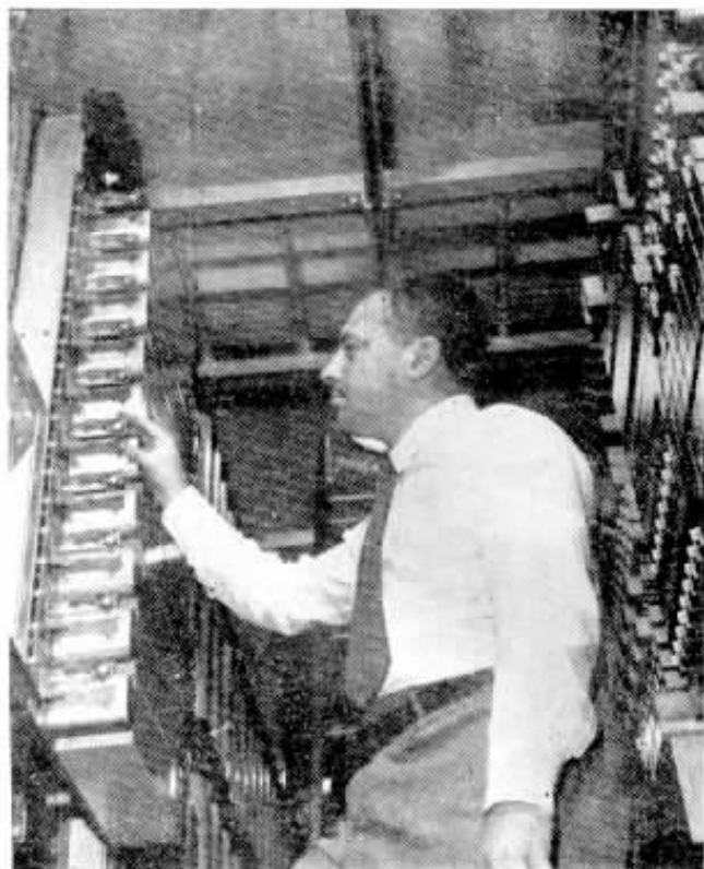
Abaixo: Raul E. Rangel, chefe do Distrito B-2, da Rede, diante do circuito de sinalização do novo aparelhamento.
