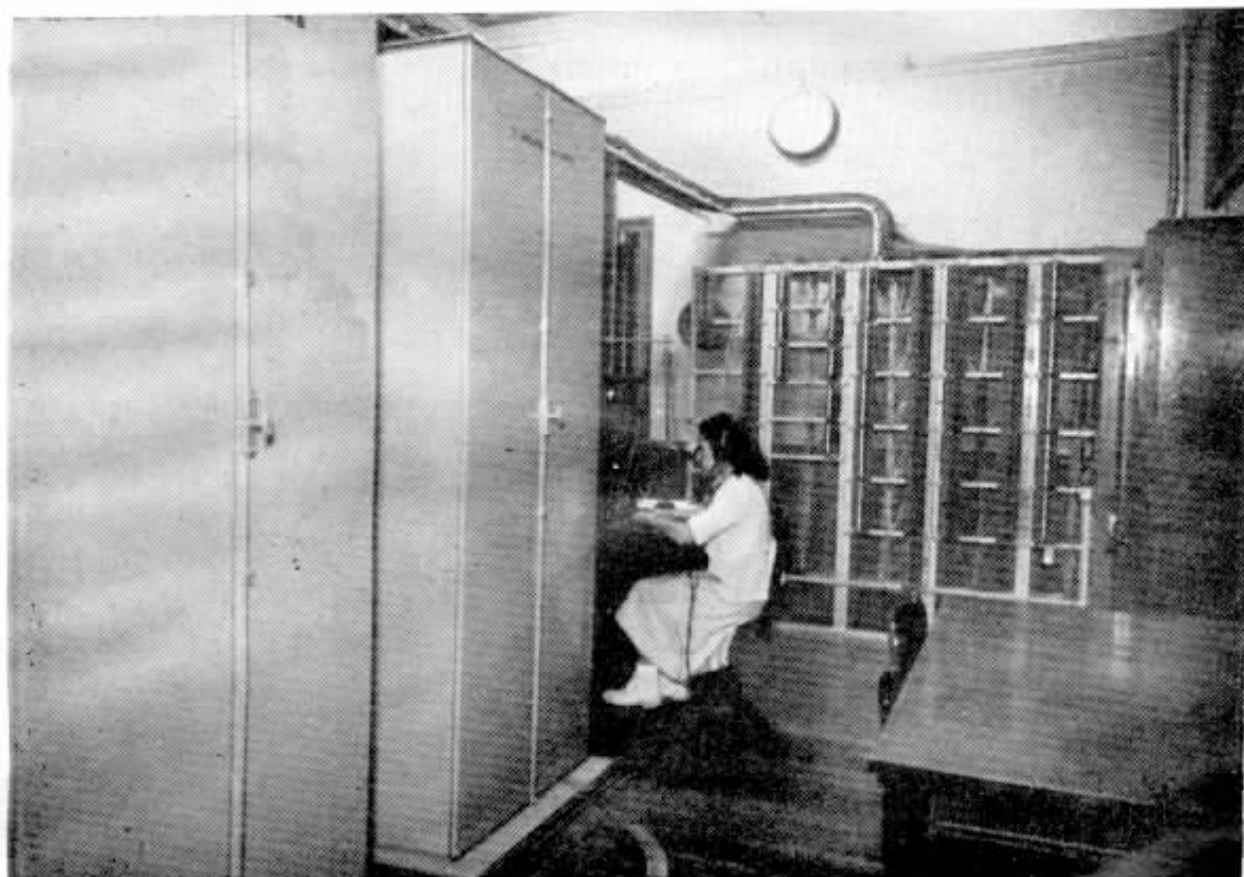
Vistas do equipamento manual e automático, no dia de sua volta ao serviço
