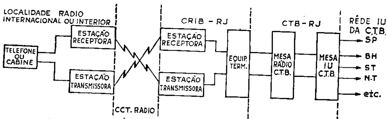
- FIG 3 - ESQUEMÁTICO DE UMA LIGAÇÃO RÁDIO INTERNACIONAL OU RÁDIO INTERIOR PARA A REDE IU DA C.T.B
