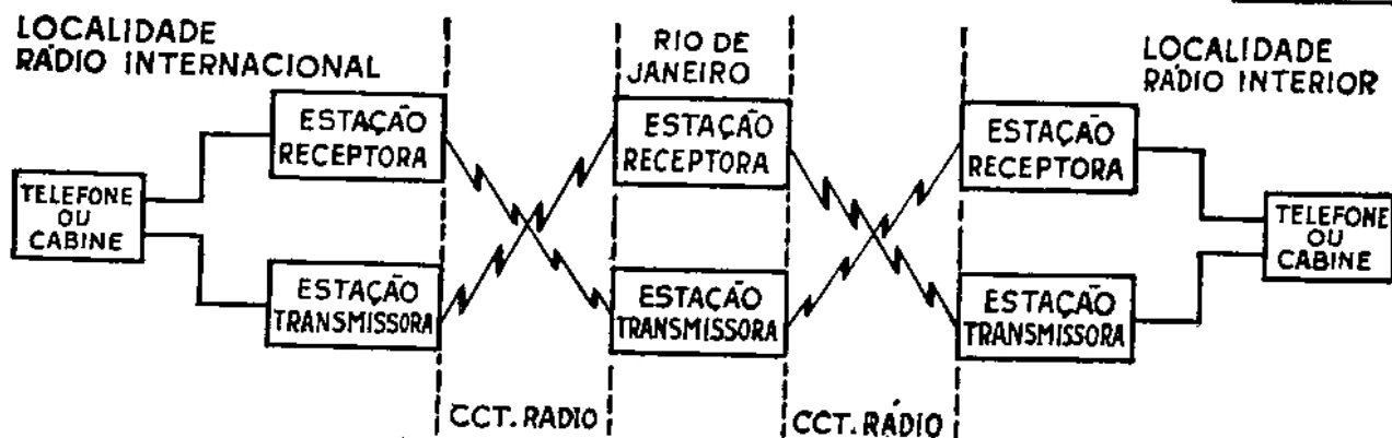
- FIG. 2 - ESQUEMÁTICO DE UMA LIGAÇÃO RÁDIO INTERNACIONAL PARA RÁDIO INTERIOR
