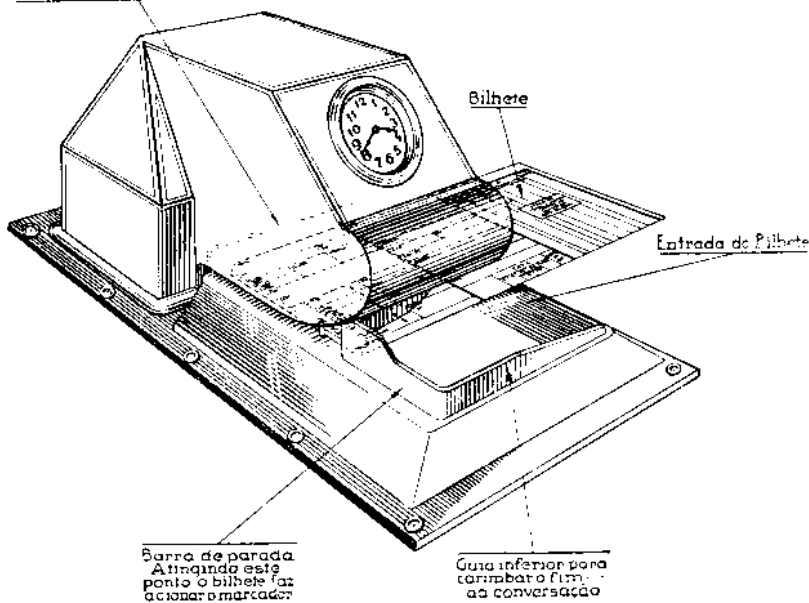
Marcador de tempo "Stromberg" automático, usado em S. Paulo e Campinas.
